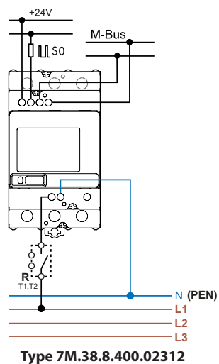
Système Modbus ou M-Bus
