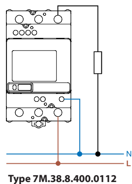
Système monophasé
