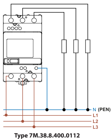
Système triphasé
