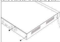
Figura 2-1 Quitar la cubierta
