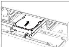
Figura 2-9 Introducir el disco duro
