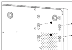
Figura 2-3 Fijar el disco duro
