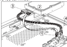
Figura 2-2 Conectar el cable
