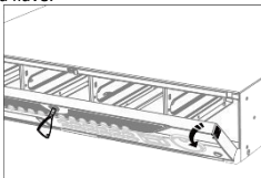
Figura 2-8 Abrir el panel frontal
