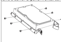
Figura 2-7 Fijar el soporte de montaje
