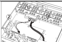
Figura 2-6 Conectar el cable
