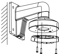
Figura 2-14 Fijar la base al soporte de montaje
