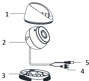
Figura 1-1 Tipo I Descripción Cámara Domo
