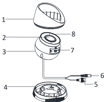
Figura 1-3 Tipo III Cámara domo Descripción
