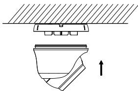
Figura 2-5 Montar el cuerpo de la cámara
