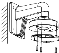
Figura 2-14 Fijar la base al soporte de montaje
