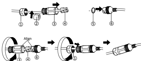
Figura 2-15 Fijar el conector de protección impermeable
