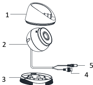
Figura 1-1 Tipo I Cámara domo Descripción
