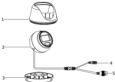
Figura 1-4 Cámara domo Descripción
