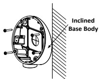
Figura 2-12 Fijar el cuerpo de la base inclinada al techo/la pared
