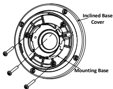
Figura 2-11 Fijar la base
