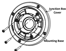
Figura 2-8 Fijar la base
