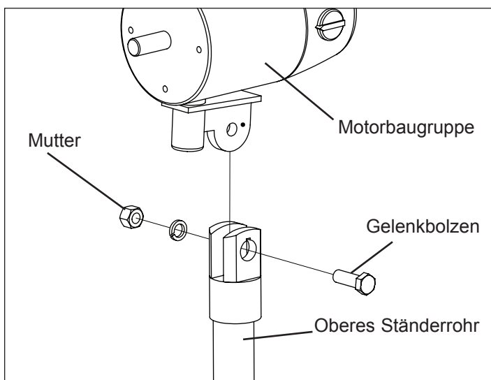
Abbildung 1: Motor an der Motorträgerbaugruppe befestigen
