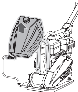
Rüttelplatte mit optionalem Wassersprühsystem
