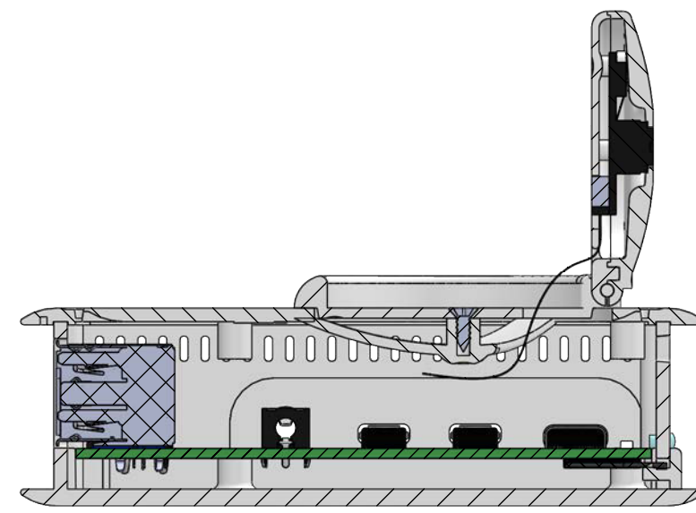
SEZIONE A-A
