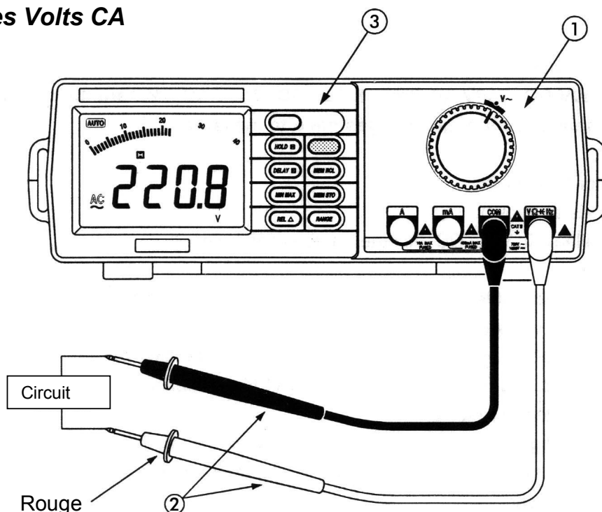
Figure 2-2. Mesures des volts CA
