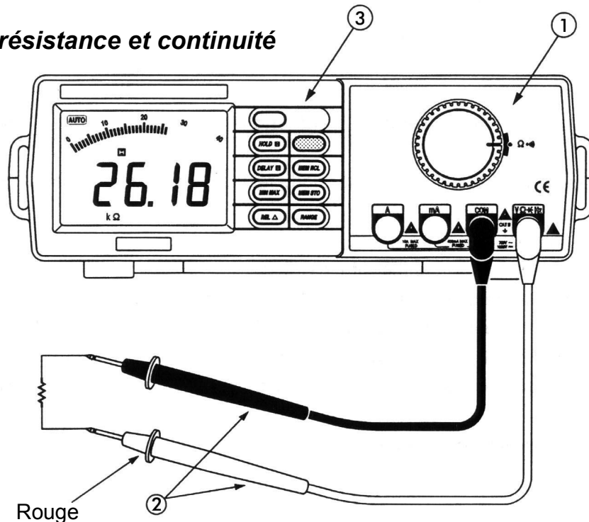
Figure 2-8. Mesures de la résistance et continuité
