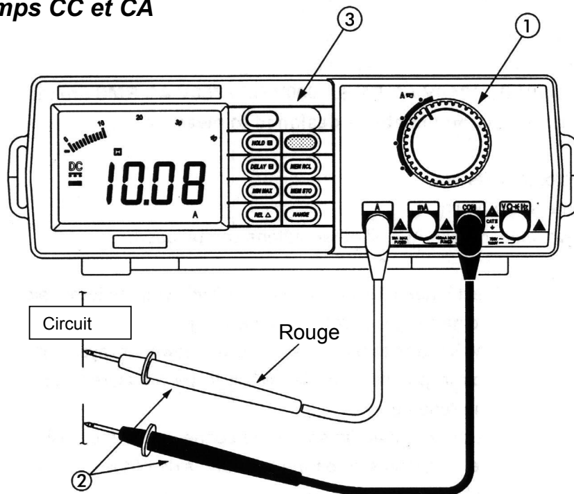
Figure 2-3. Mesure des Amps
