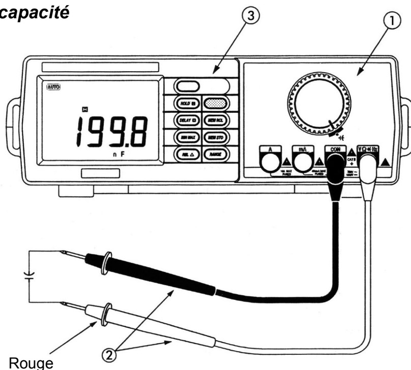
Figure 2-6. Mesures de capacité
