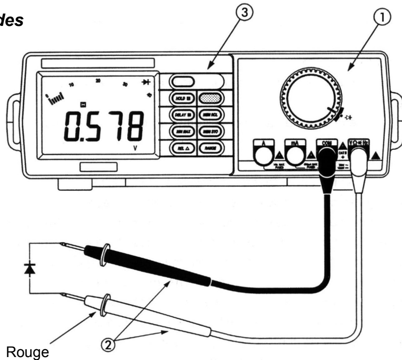
Figure 2-7. Test des diodes
