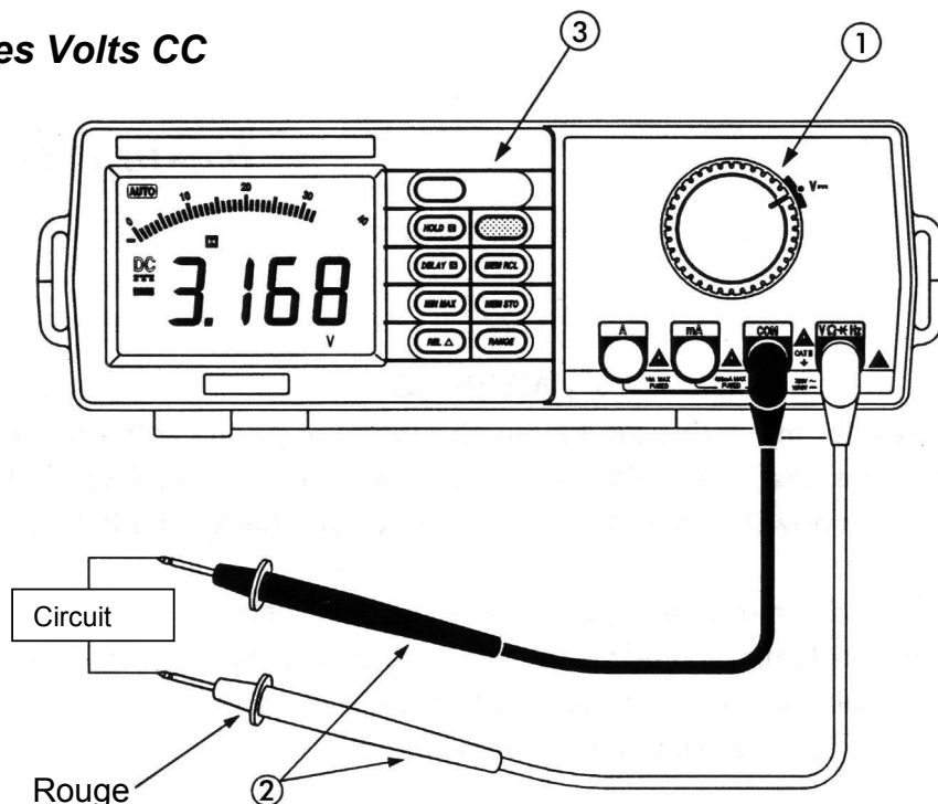
Figure 2-1. Mesures des Volts CC
