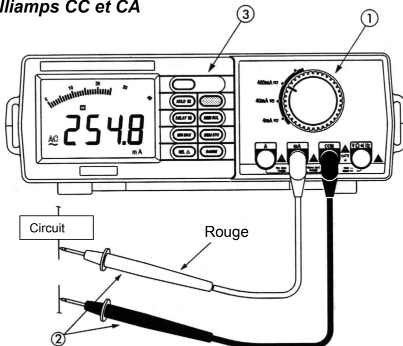
Figure 2-4. Mesures des milliamps
