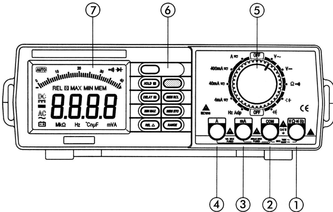
Figure 1-1. Caractéristiques du multimètre de table (Avant)
