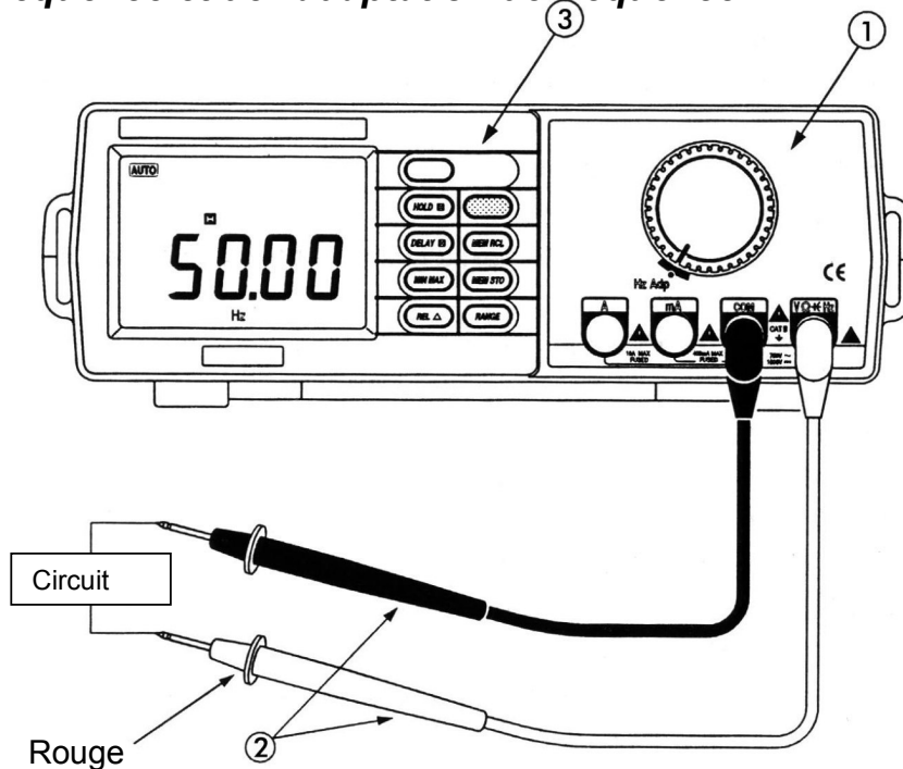
Figure 2-5. Mesure de la fréquence et de l'adaptation de fréquence (ADP)
