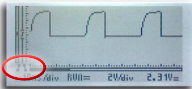
Pendiente ascendente
